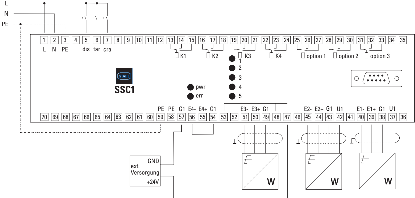
Relaiszuordnung Modus 1-2-3
