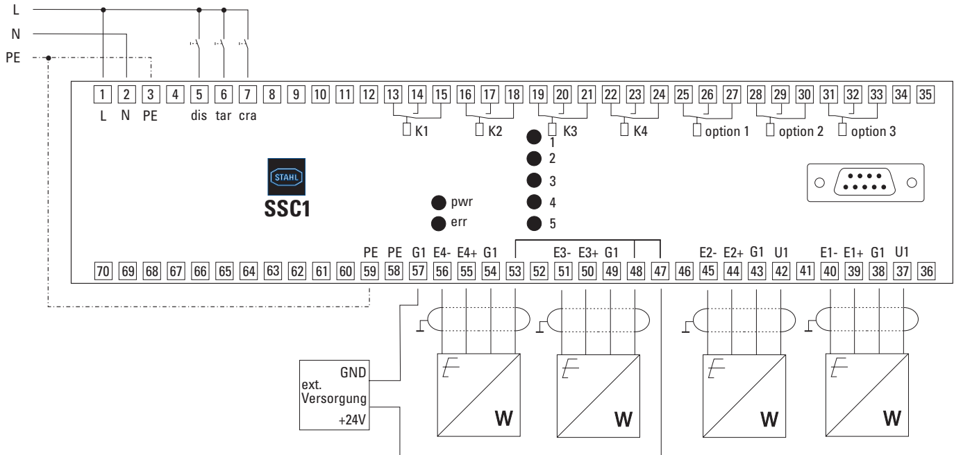
Prinzipschaltbild SSC1
