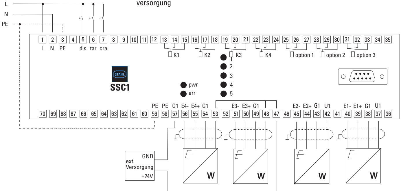
Relaiszuordnung Modus 6-4-4
