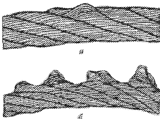
Рис. 12. Выдавливание проволок прядей: a — в одной пряди; б — в нескольких прядях
