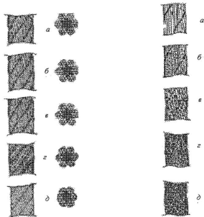
Рис. 5. Износ наружных проволок каната крестовой свивки:
