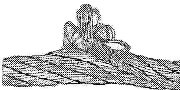
Рис. 11. Выдавливание сердечника
