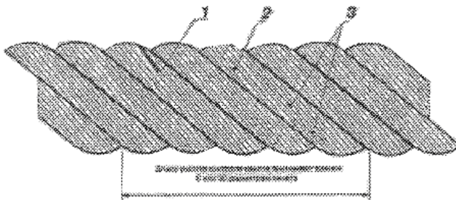
Рис. 4. Пример определения числа обрывов наружных проволок стального каната 1 – на участке контроля у оборванной проволоки обнаружен только один конец, ответный конец оборванной проволоки отсутствует. Данный дефект соответствует одному обрыву; 2 – на участке контроля у оборванной проволоки в наличии два конца. Данный дефект соответствует одному обрыву; 3 – на участке контроля одна из проволок имеет двукратное нарушение целостности. Поскольку нарушение целостности принадлежит только одной проволоке, данный дефект суммарно соответствует одному обрыву.
