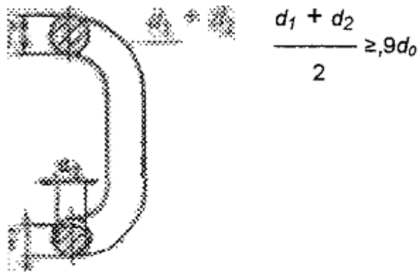
Рис 2. Уменьшение диаметра сечения звена цепи:
