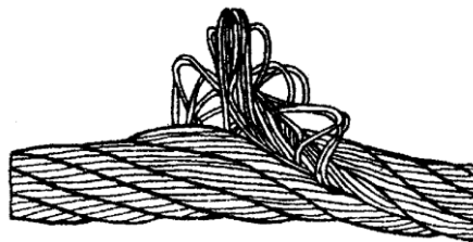
Рис. 11. Выдавливание сердечника
